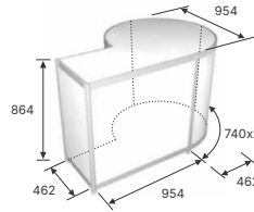
Stalas - baras Bar table
